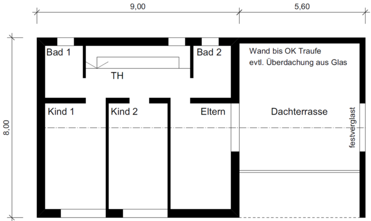
Obergeschoß
